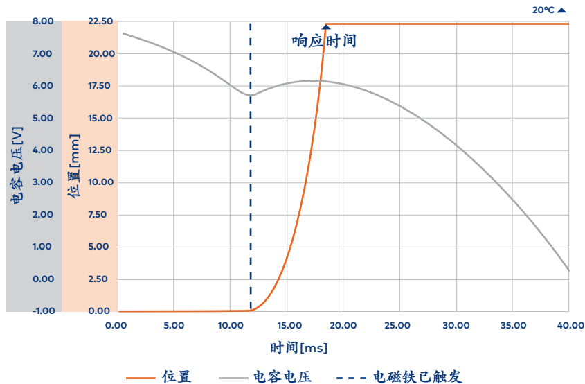
20°C 电容放电 (1000 mF)
